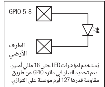
Q-SYS مؤشر LED الذي يعمل بطاقة
