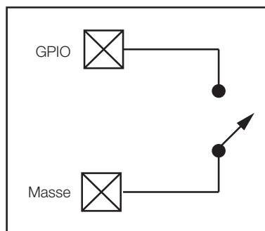
Schalter- oder Kontaktschluss
